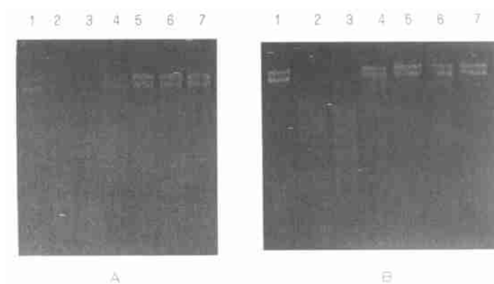
图2 EDTA处理后螺旋藻胞内核酸酶对 pEUTISI 的降解作用
