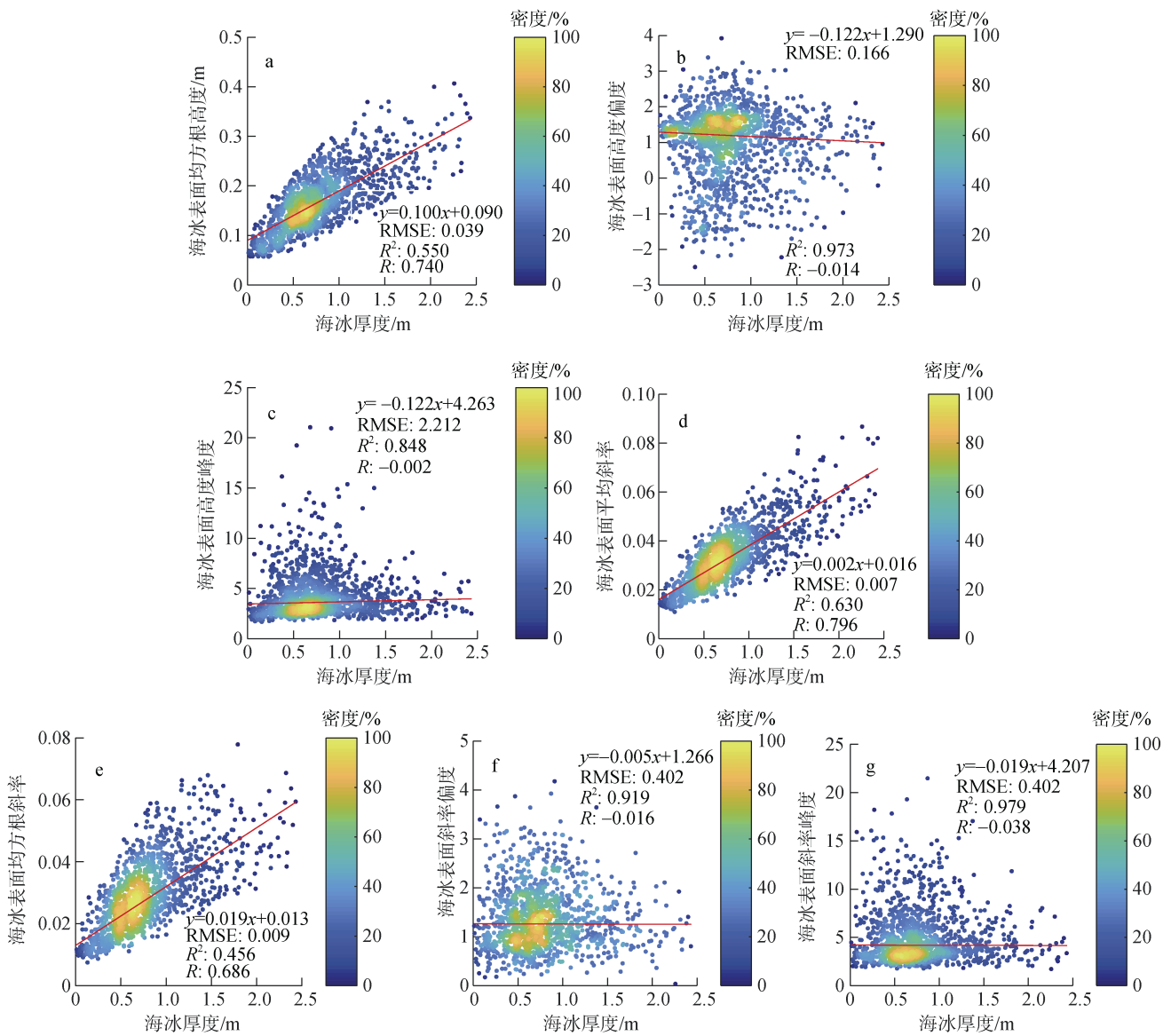
图 3 海冰厚度与海冰表面粗糙度参数的散点图以及线性回归模型及拟合效果
