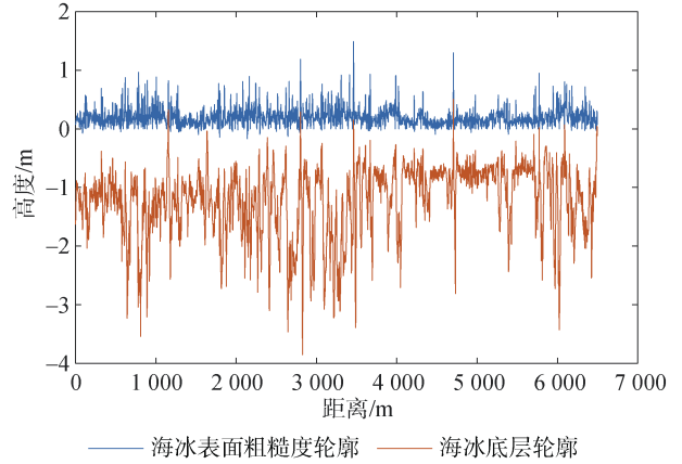
图 2 2011 年 3 月 20 日拉布拉多海的海冰的表面粗糙度(上线)和冰吃水(下线)剖面图示例
