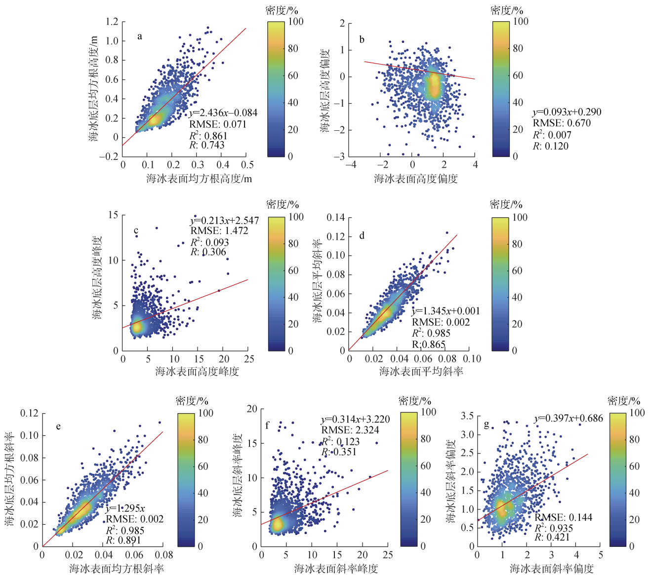
图 7 海冰表面和底层粗糙度的散点图以及线性回归模型及拟合效果
