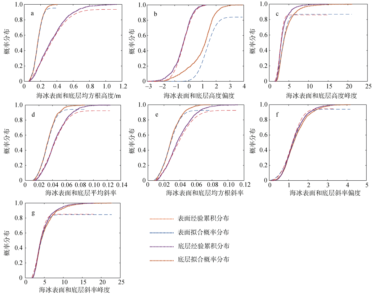
图 6 海冰表面和底层各粗糙度参数的累积概率分布曲线
