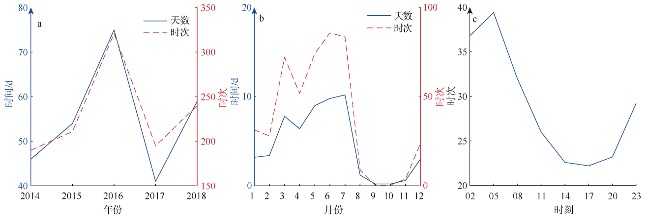
图 2 2014—2018 年海雾天数和次数变化曲线
