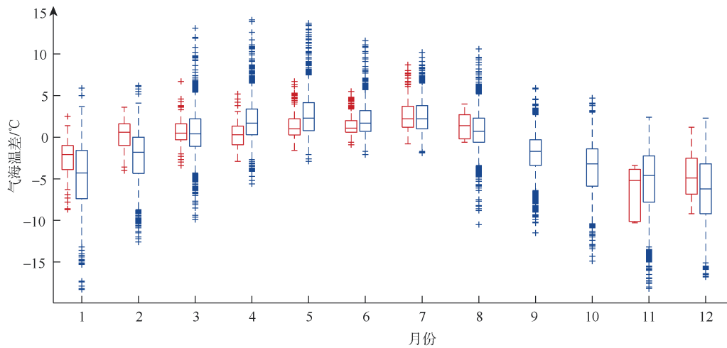
图 3 逐月气海温差分布盒须图
