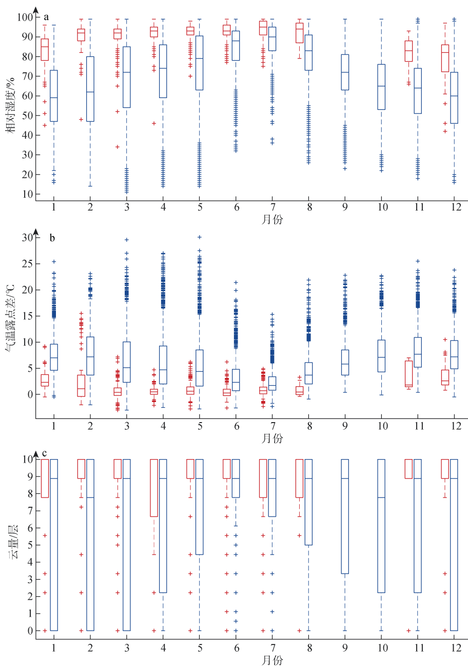
图 4 逐月相对湿度(a)、气温露点差(b)和云量(c)分布盒须图
