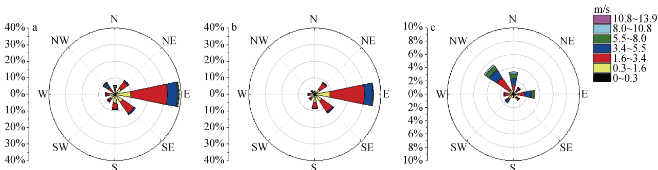
图 5 海雾发生时次海面风玫瑰图 Fig. 5 Wind rose charts for sea fog cases 注: a: 全年; b: 3—9 月; c: 1、2、12 月
