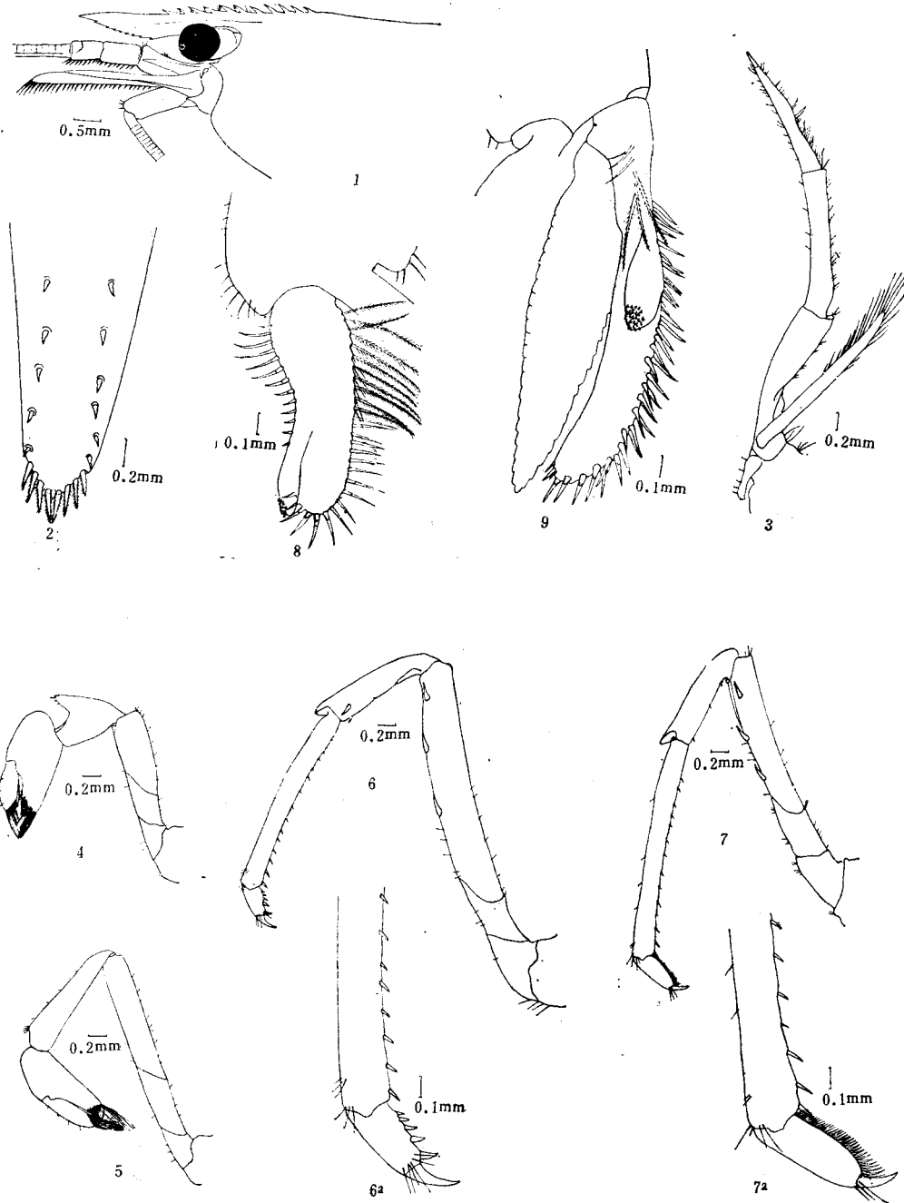
图 3 长棍米虾(新种) Caridina longa sp. nov.
