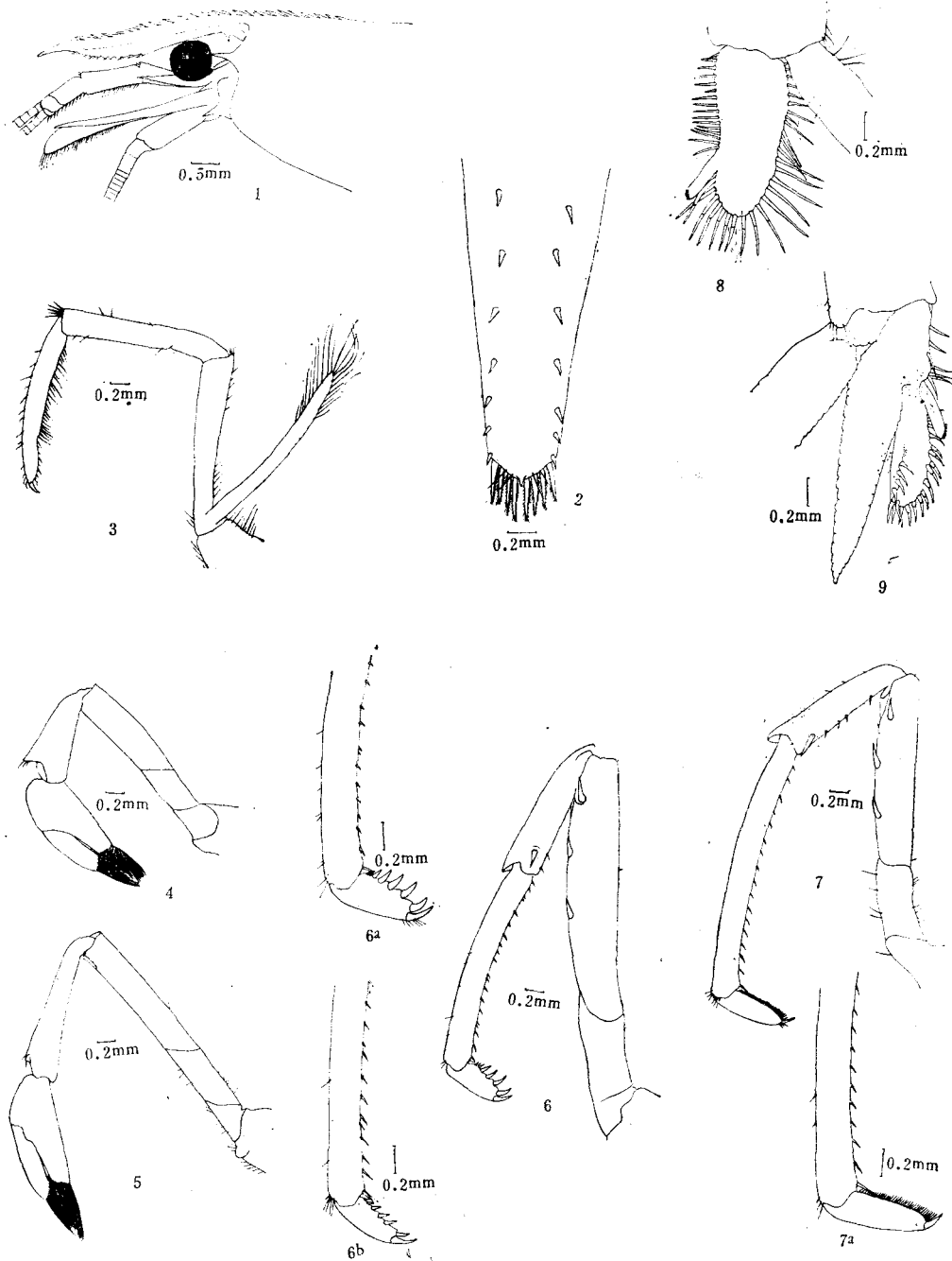
图 2 异指米虾(新种) Caridina heterodactyla sp. nov.
