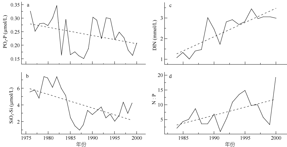
图5 南黄海表层水体 \text{PO}_4\text{-P} 、 \text{SiO}_3\text{-Si} 、DIN 和 N:P 的年度变化(引自 Lin 等(2005))
