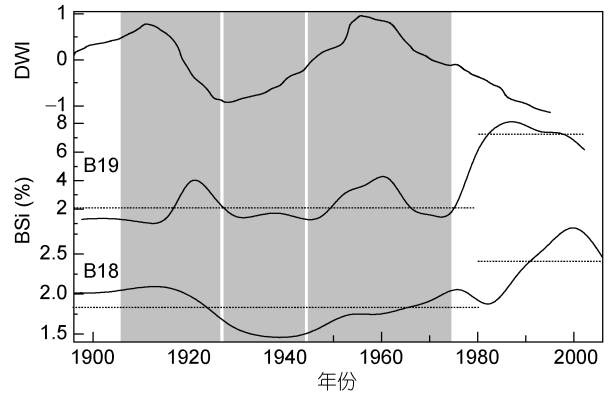
图4 南黄海近海上覆水初级生产力(沉积物 BSi)和华北平原及邻近地域干湿指数(DWI)的年代际波动趋势
