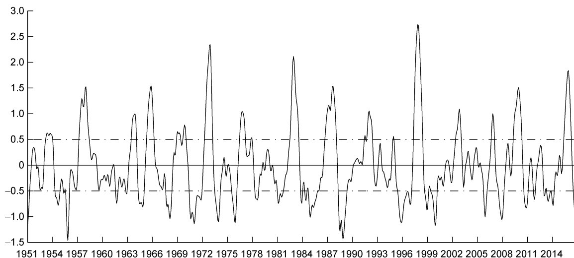
图 3 1951 年 1 月至 2016 年 9 月的 Niño3.4 指数时间序列 Fig.3 Time Series of Niño3.4 index from January 1951 to September 2016
