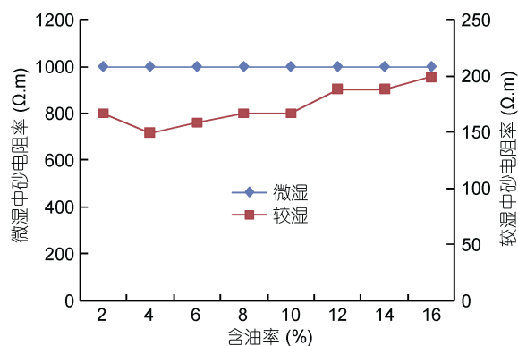
图 8 含油率对中砂电阻率的影响
