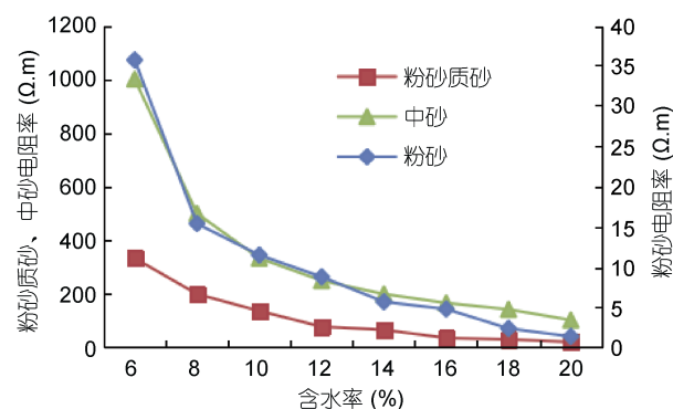
图 2 不同含水率的未污染沉积物电阻率
