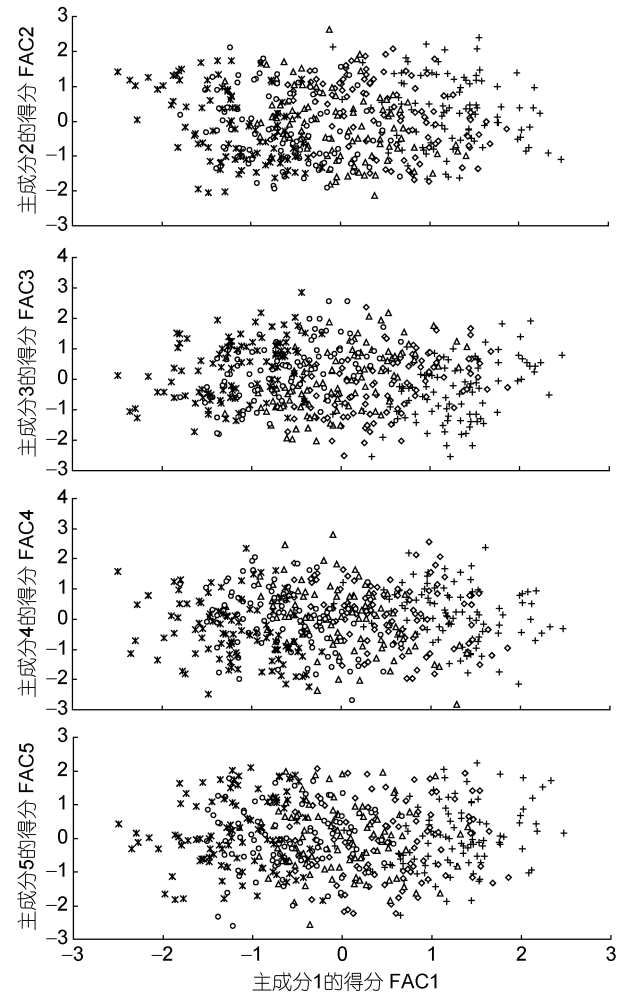
图 2 主成分散布图
