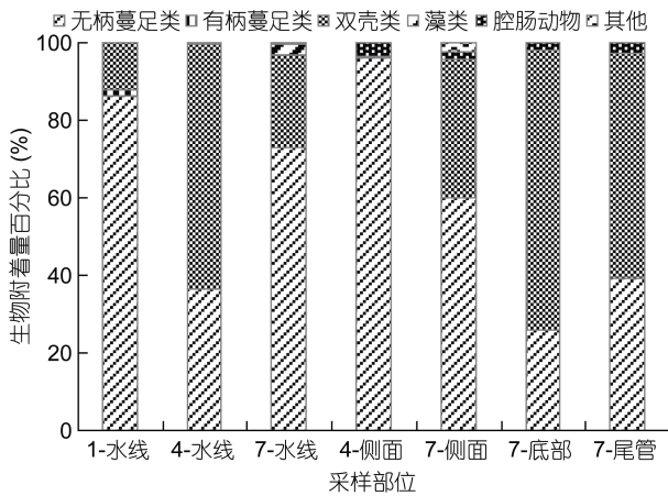
图3 雷州半岛东部近海浮标大型固着生物附着量的百分比组成
