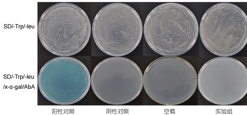
图4 pGBKT7- PyMAPK5 诱饵蛋白自激活检测
