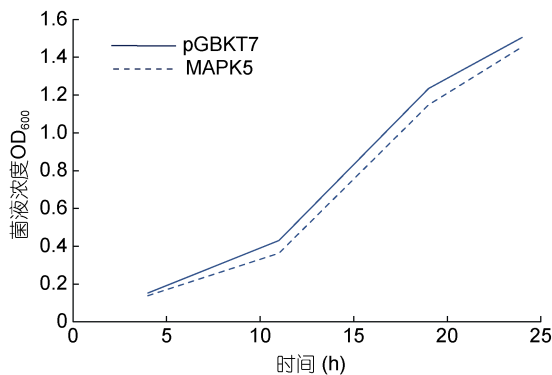
图5 pGBKT7- PyMAPK5 诱饵蛋白毒性检测
