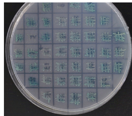
图6 PyMAPK5 筛选得到的阳性克隆
