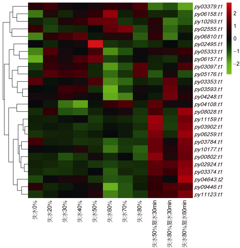
图 9 PyMAPK5 互作蛋白基因失水胁迫下表达谱分析
