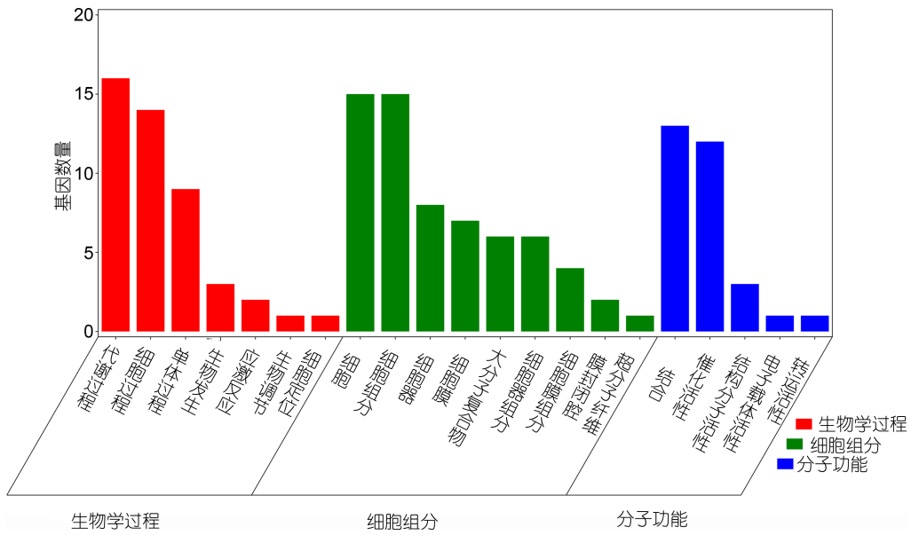
图 8 PyMAPK5 候选互作蛋白 GO 注释
