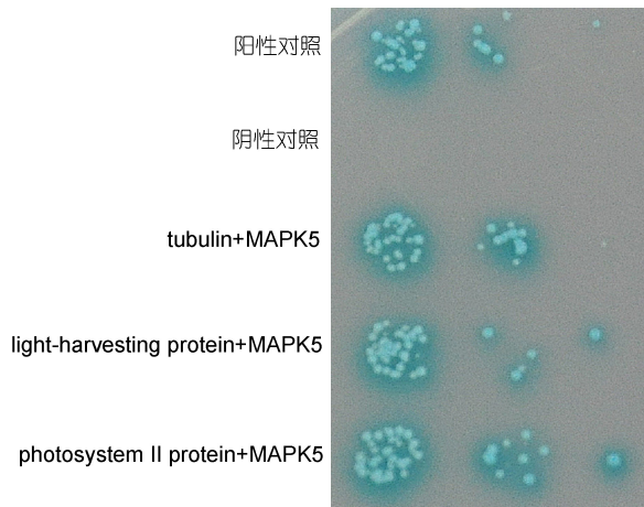
图 10 PyMAPK5 候选互作蛋白 SD/-Trp/-Leu /-His/-Ade/x- \alpha -gal/AbA 培养基一对一验证
