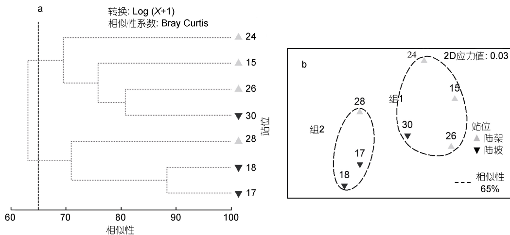
图 4 基于南海北部 7 个站位小型底栖动物类群丰度矩阵的聚类(a)和排序分析(b)
