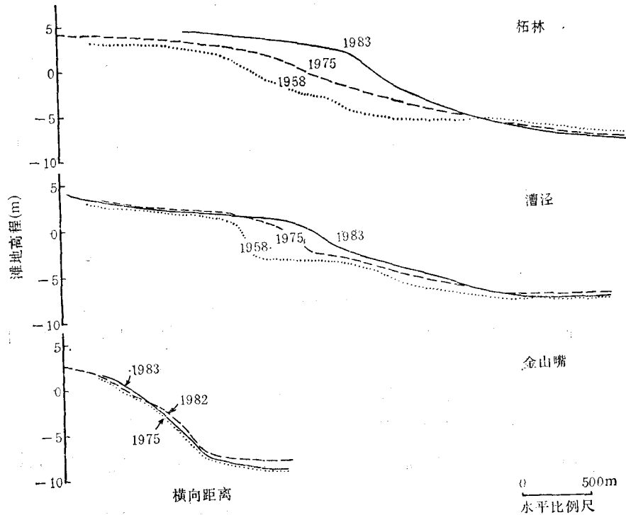
图5 潮滩冲淤对比图
