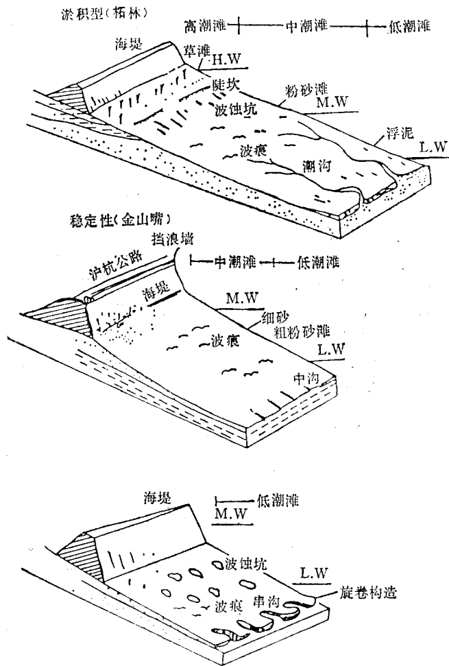
图4 潮滩地貌类型断块图
