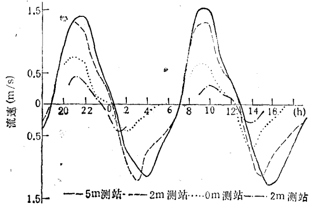
图9 柘林潮滩流速过程线对比
