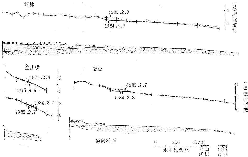
图10 潮滩冲淤和沉积剖面图
