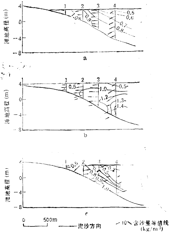
图 7 潮滩剖面悬沙分布
