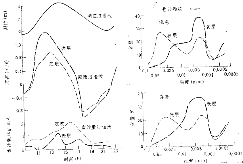
图 8 金山嘴表、底层流速和含沙量过程线图
