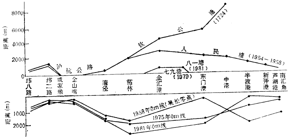
图 3 潮滩 0m 线与海堤距离的变化图
