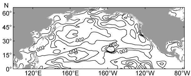
图 12 北太平洋风速变化趋势的空间分布(单位: m/a)
