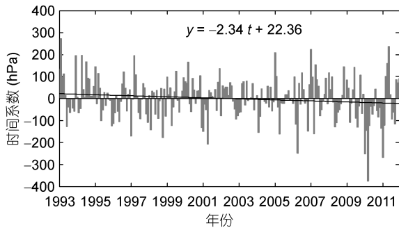
图 10 北大西洋 SLP 时间系数(第一模态)的变化趋势
