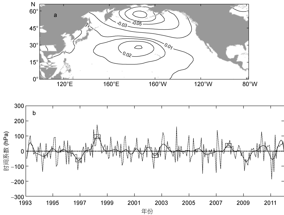
图 16 SLP 第二模态的空间分布(a)及对应的时间系数(b)
