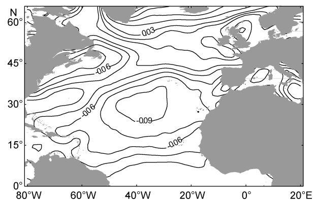
图 5 北大西洋 SLP 变化趋势的空间分布(单位: hPa/a) Fig.5 Spatial distribution of SLP trend in North Atlantic (unit: hPa/a)
