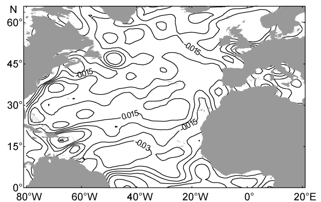
图 4 北大西洋风场变化趋势的空间分布(单位: m/a) Fig.4 Spatial distribution of wind trend in North Atlantic (unit: m/a)
