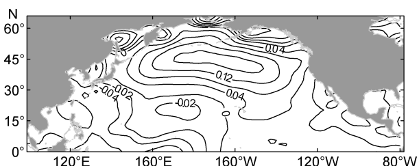
图 13 北太平洋 SLP 变化趋势的空间分布(单位: hPa/a)
