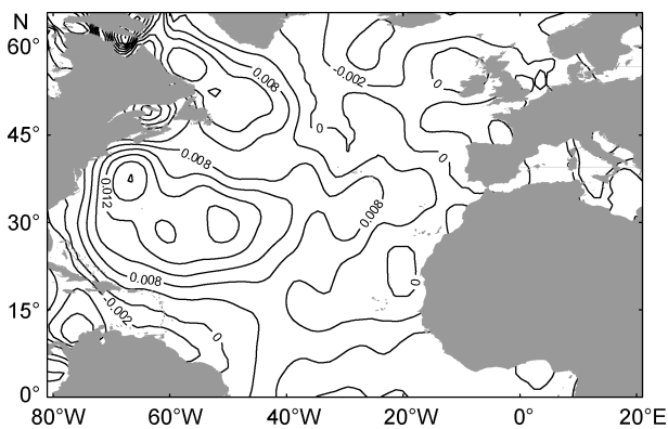
图 3 北大西洋波浪变化趋势的空间分布(单位: m/a) Fig.3 Spatial distribution of wave trend in North Atlantic (unit: m/a)
