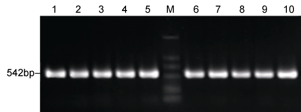
图 1 紫扇贝和海湾扇贝 16S rDNA 基因片段的 PCR 扩增产物
