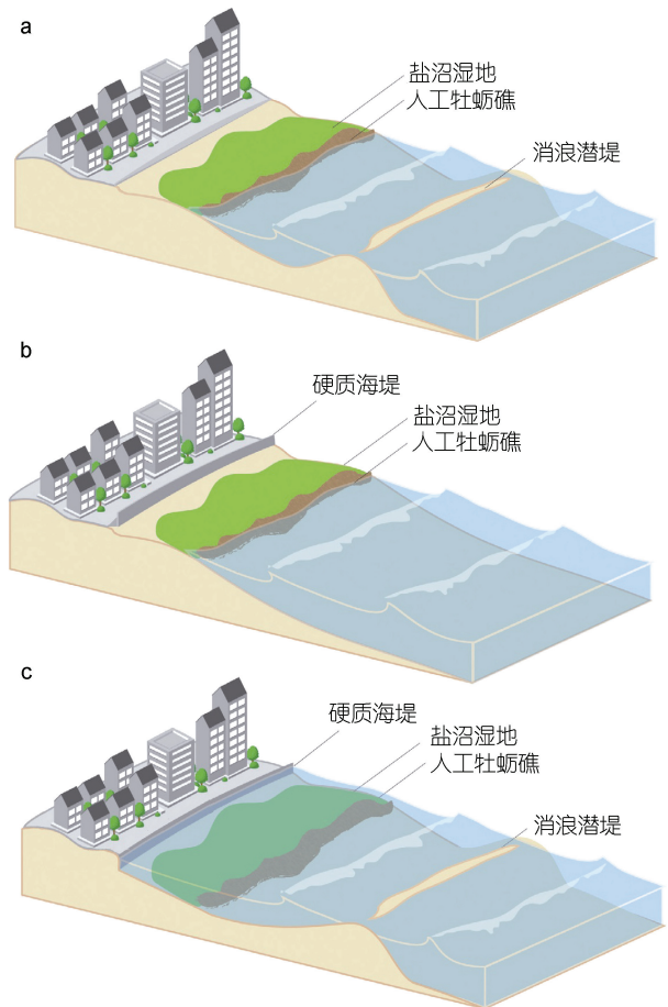
图 1 生态海岸防护工程示意图 (修改自 Sutton-Grier et al. , 2015)
