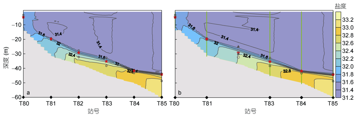
图 4 经过深度坐标变换处理后得到的盐度断面分布(资料同图 2)
