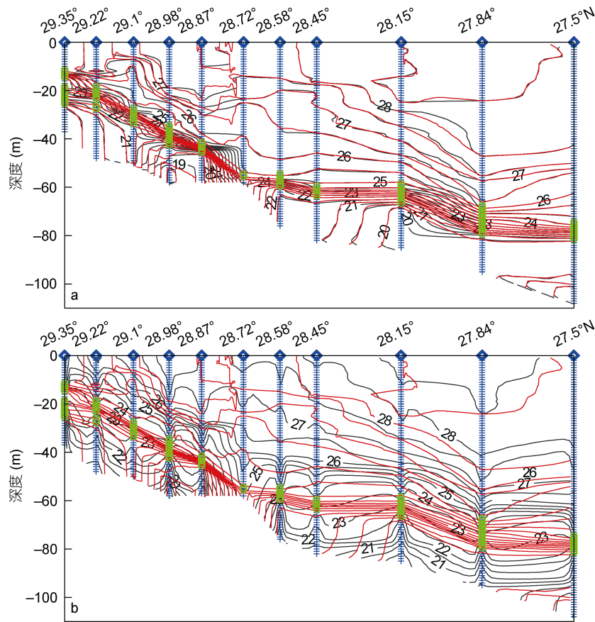
图 6 8 月初舟山东南海陆架海域的一条观测断面的温度分布
