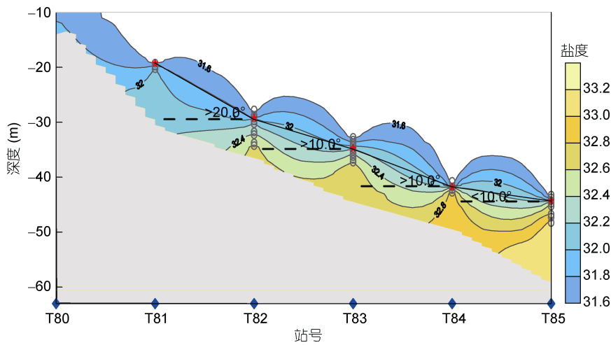
图3 图 2a 盐度断面分布图中盐跃层特征提取示意图
