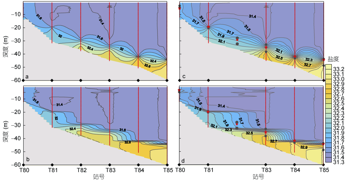
图2 泰国湾内的一条盐度断面分布图
