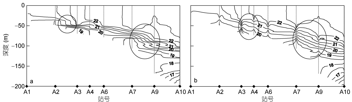
图 1 南海北部一断面盐度分布图
