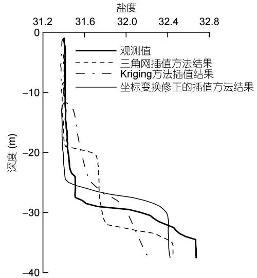
图 5 T82 测站处盐度观测值及图 2c 和 d、图 4b 中盐度插值结果的垂向分布
