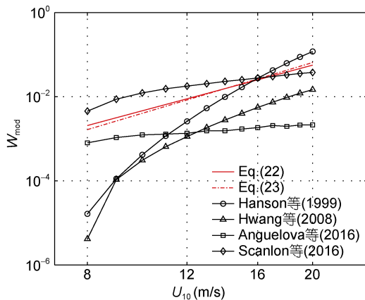
图 7 其他研究者的参数化方案与式(22)、式(23)对比 Fig.7 Comparison in the parameterization among other authors', Eq.(22), and Eq.(23)
