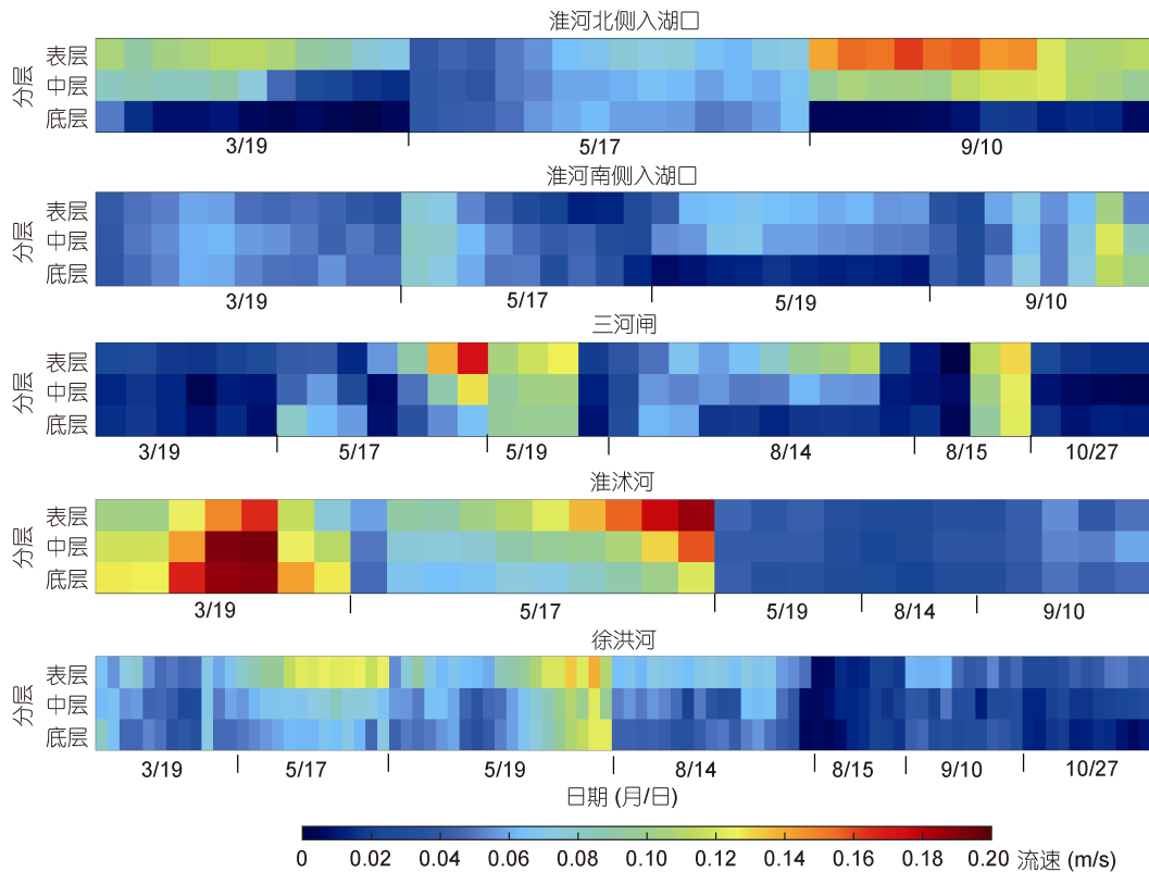
图 6 洪泽湖 5 条主要入湖河道分层水体流速
